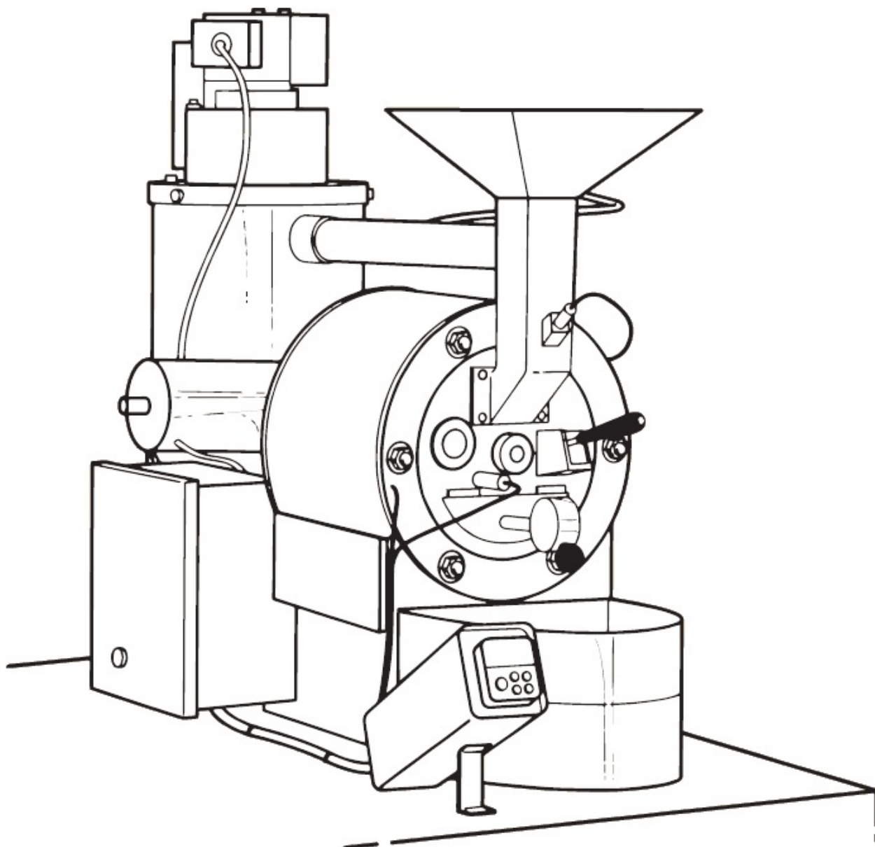
Ростер рис
