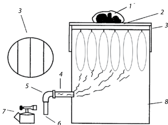
Рис. 7. Коптильня с пеналом, приваренным к стенке бочки:
