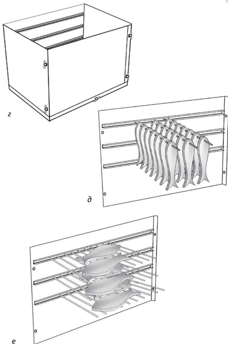
Рис. 4. Походная коптильня горячего копчения:
