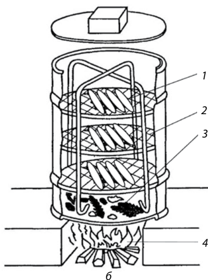
Рис. 9. Коптильня горячего копчения из металлической бочки: а — вариант с решетками на раме, опирающейся на дно бочки; б — вариант с подвешенной решеткой: 1 — рыба; 2 — решетка; 3 — противень; 4 — топка
