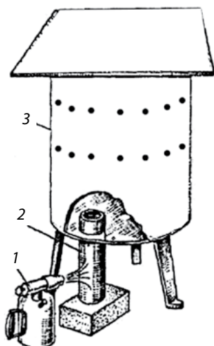
Рис. 8. Коптильня с пеналом, вкрученным в днище бочки:
