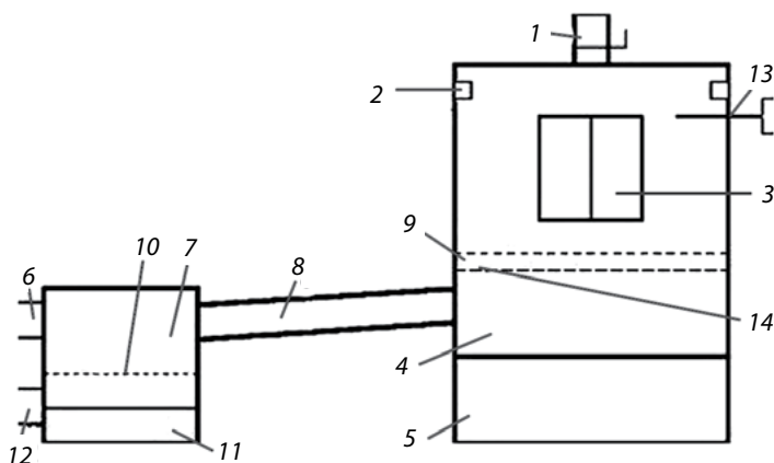
Рис. 11. Установка холодного копчения:
