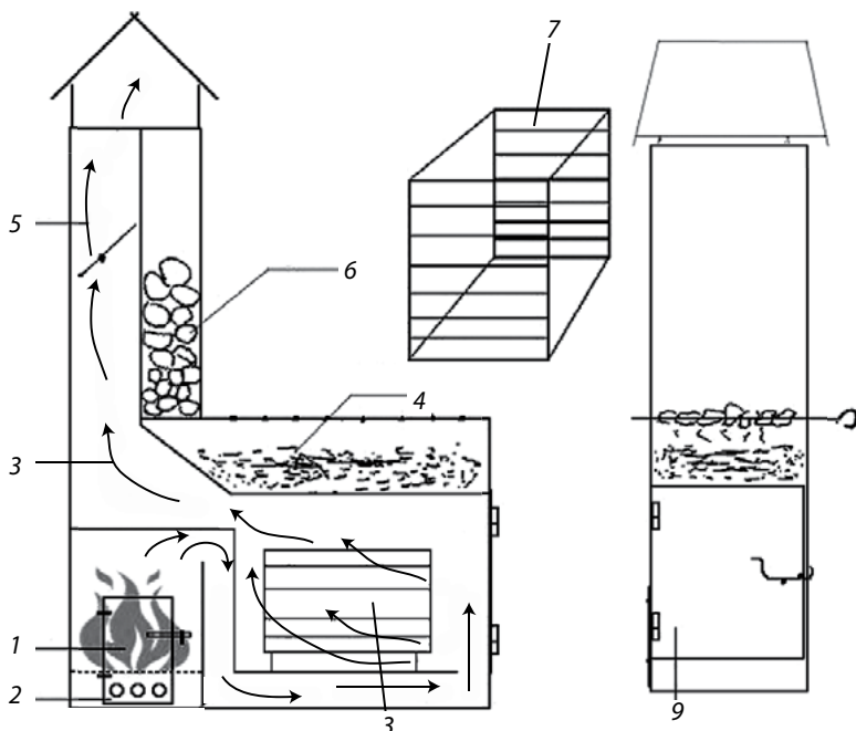
Рис. 17. Схема коптильни-мангала:
