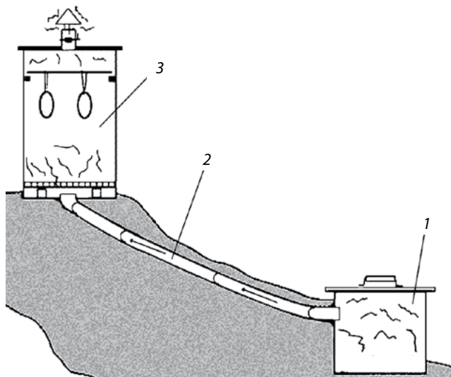
Рис. 1. Классическая конструкция коптильни для холодного копчения: 1 — дымогенератор (очаг); 2 — дымовой канал (траншея); 3 — коптильня
