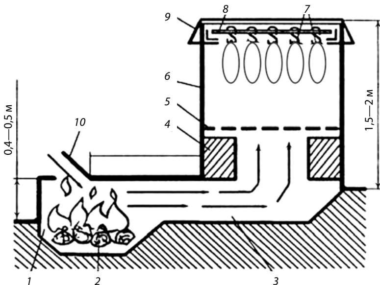
Рис. 2. Подземная коптильня простейшей конструкции:
