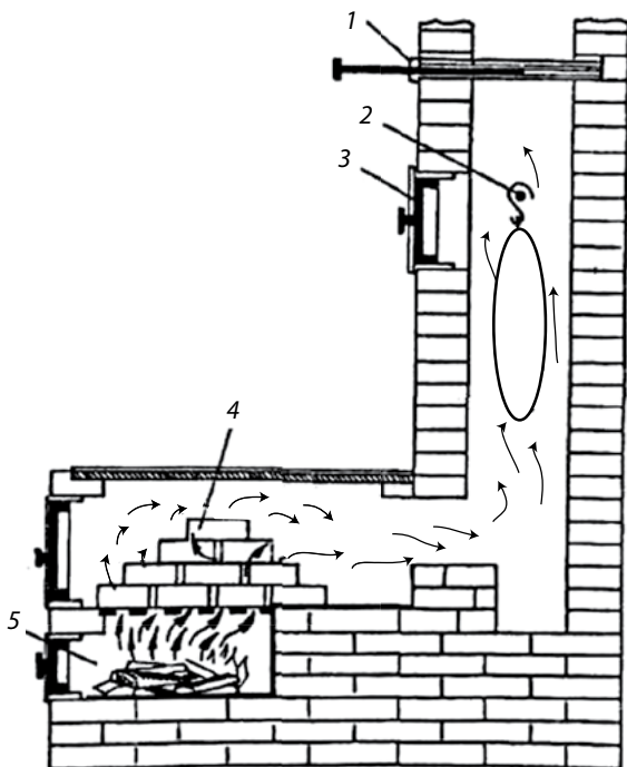
Рис. 18. Коптильня в печной дымоходной трубе:
