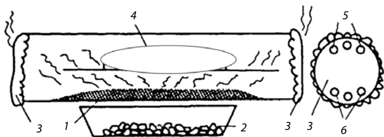
Рис. 12. Труба-коптильня:
