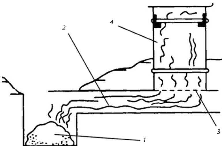
Рис. 10. Компонировочная схема установки холодного копчения:
