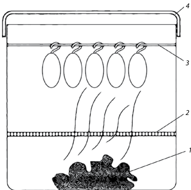
Рис. 3. Простейшая коптильня горячего копчения:
